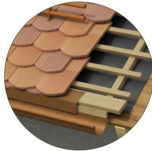
DÉTAIL 2
