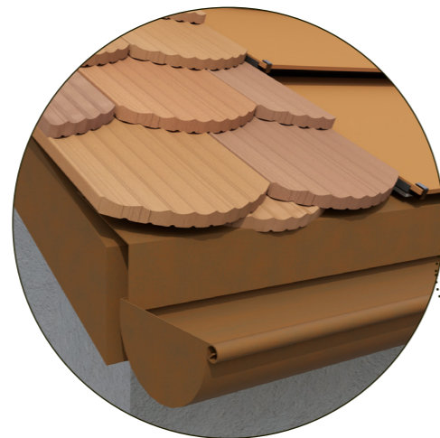
DÉTAIL 3
