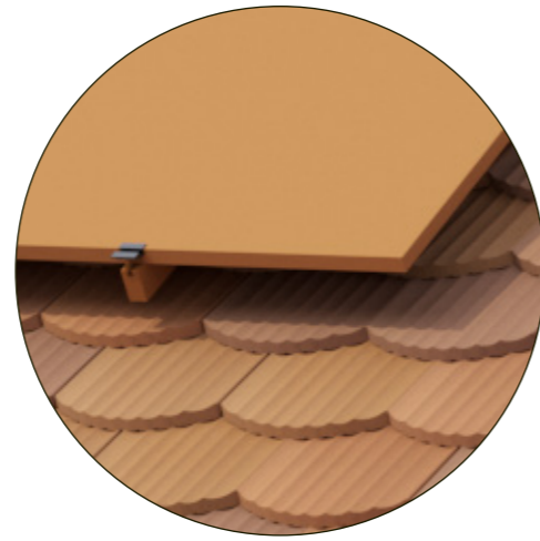
DÉTAIL 1
